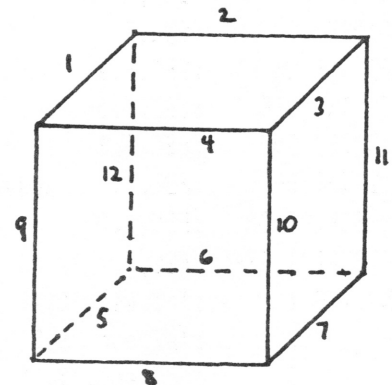
EDGE LIST
